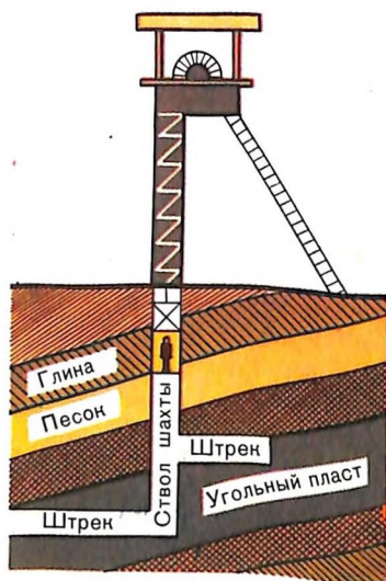
17. Шахтанын схемасы.
