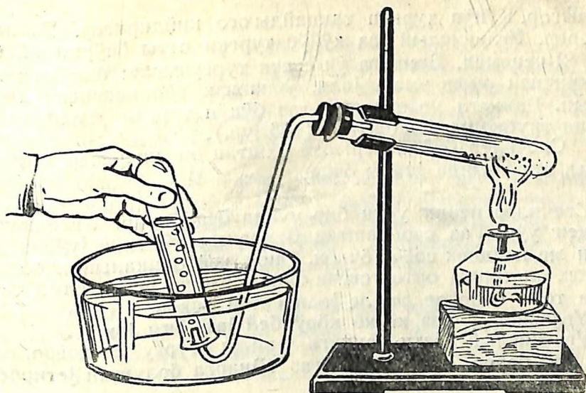
103 жүр. Кислород аларына керектү прибор.
