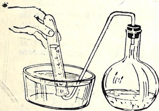
105 жүр. Углекислый газты аларына керектү прибор.
