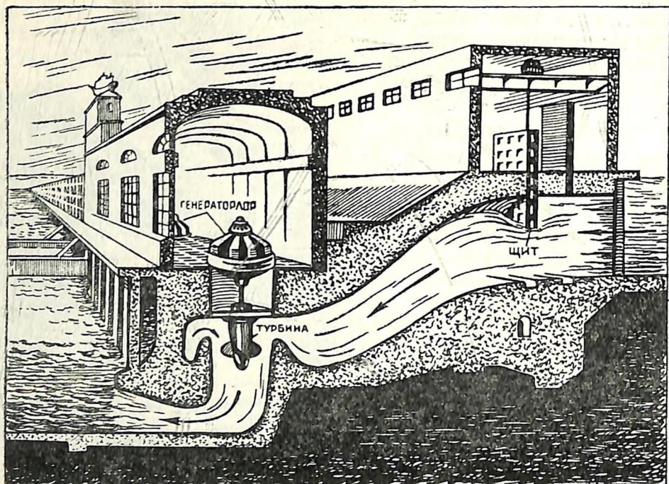
61 жур. Гидроэлектростанцияның ич жанының бұдүми.
