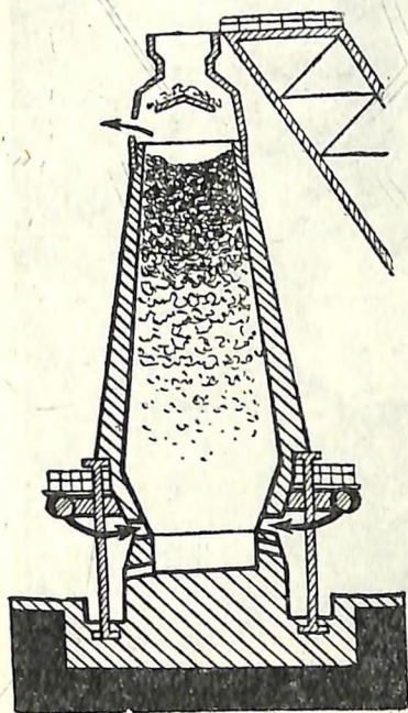
53 жүр. Доменный печке (жара кезип көргүскөни): үстүндеги стрелка — домна-дан газ чыгар жер; түбү жанында эки стрелка — домнага изү кей кирер жер; кайылып кайнап турган чойды ак өңлө көргүскөн.
