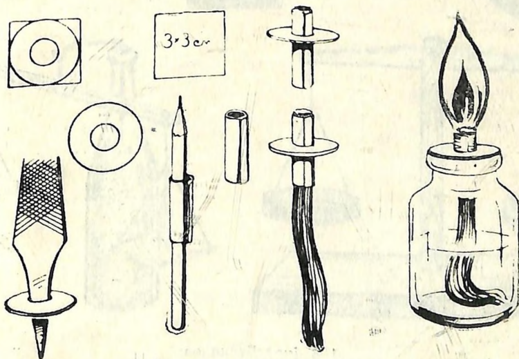
182 жүр. Спиртовканы канайда жазаары.
