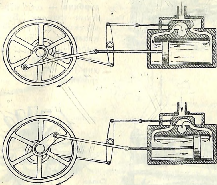
21 јур. Бууныг нйдезиле иштеер поршень канайда эдилген.
