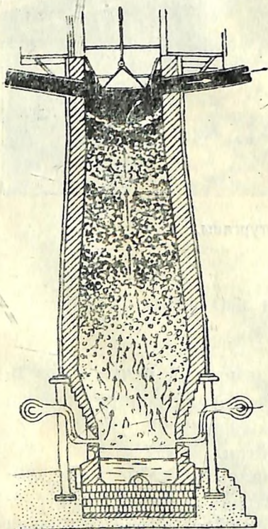
74 жүр. Доменная печь (жара кезип көргүскени).
