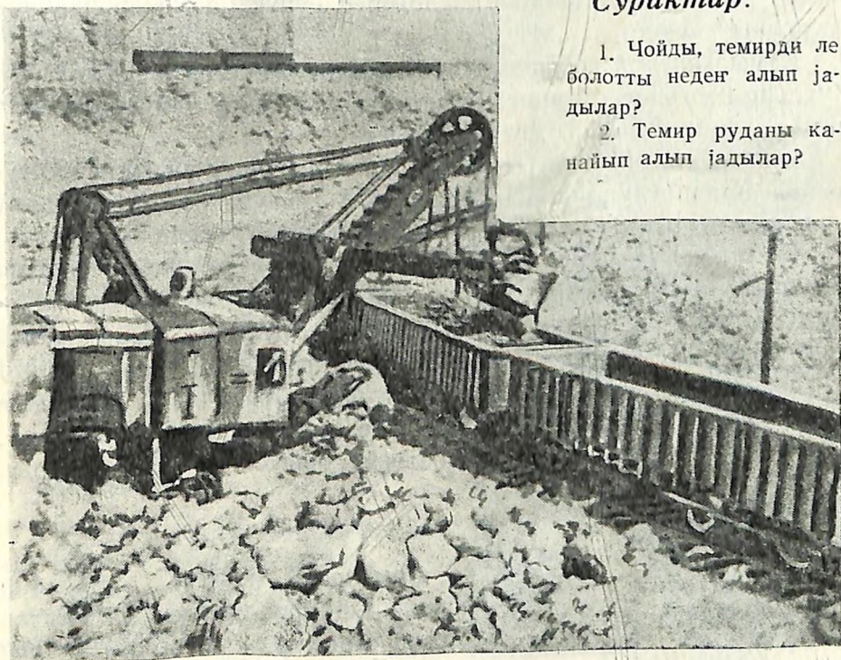
73 јур. Руданы коштоп турганы.
