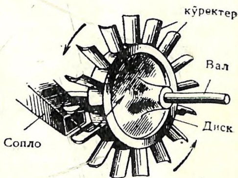
24 жур. Буунын ийдезиле иштеер турбина.
