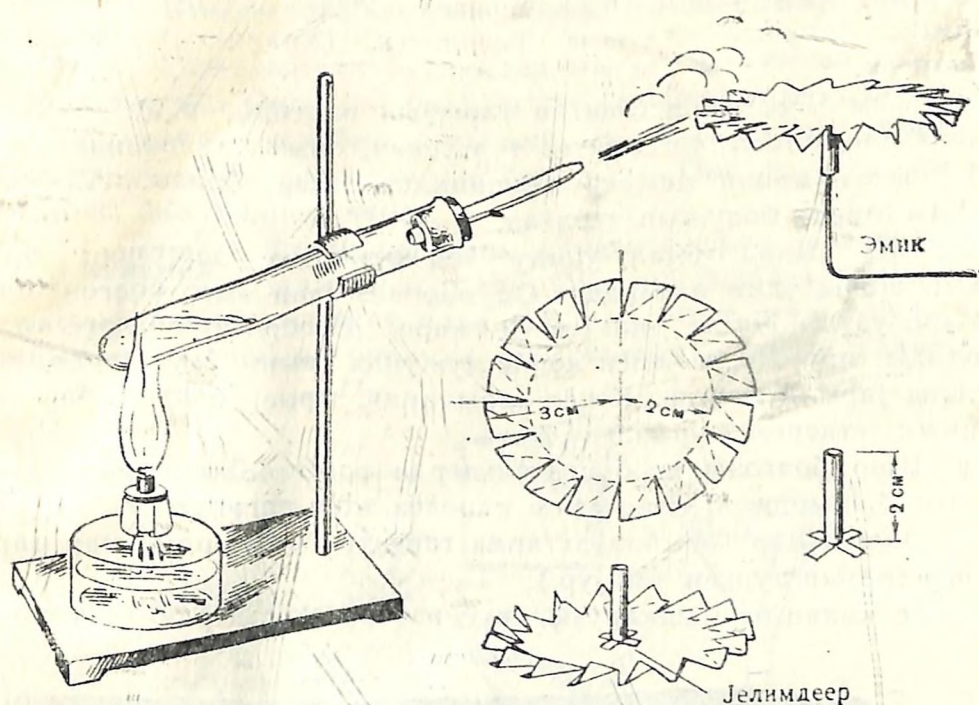
25 жүр. Буунын ийдезиле иштеер турбинанын чаазыннанг эткен модели.
