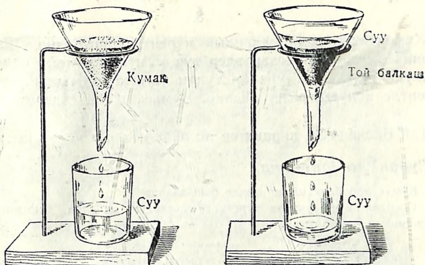
52 сур. Суу кумакты өткүрө түрген өдөт. Той балкашты дезе коомой өдүп жат.
